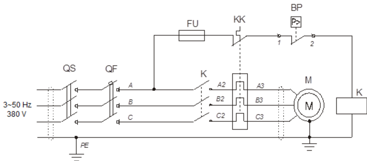
Obrázek A.1 – Schéma elektrických obvodů kompresoru F-500.LT100
